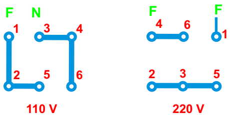
TESTE PARA VERIFICAR TENSÃO
