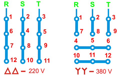
TRIFÁSICO - 12 TERMINAIS
