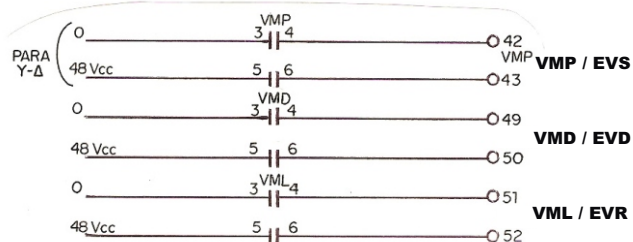
Diagrama Elétrico do Bloco de Válvulas
