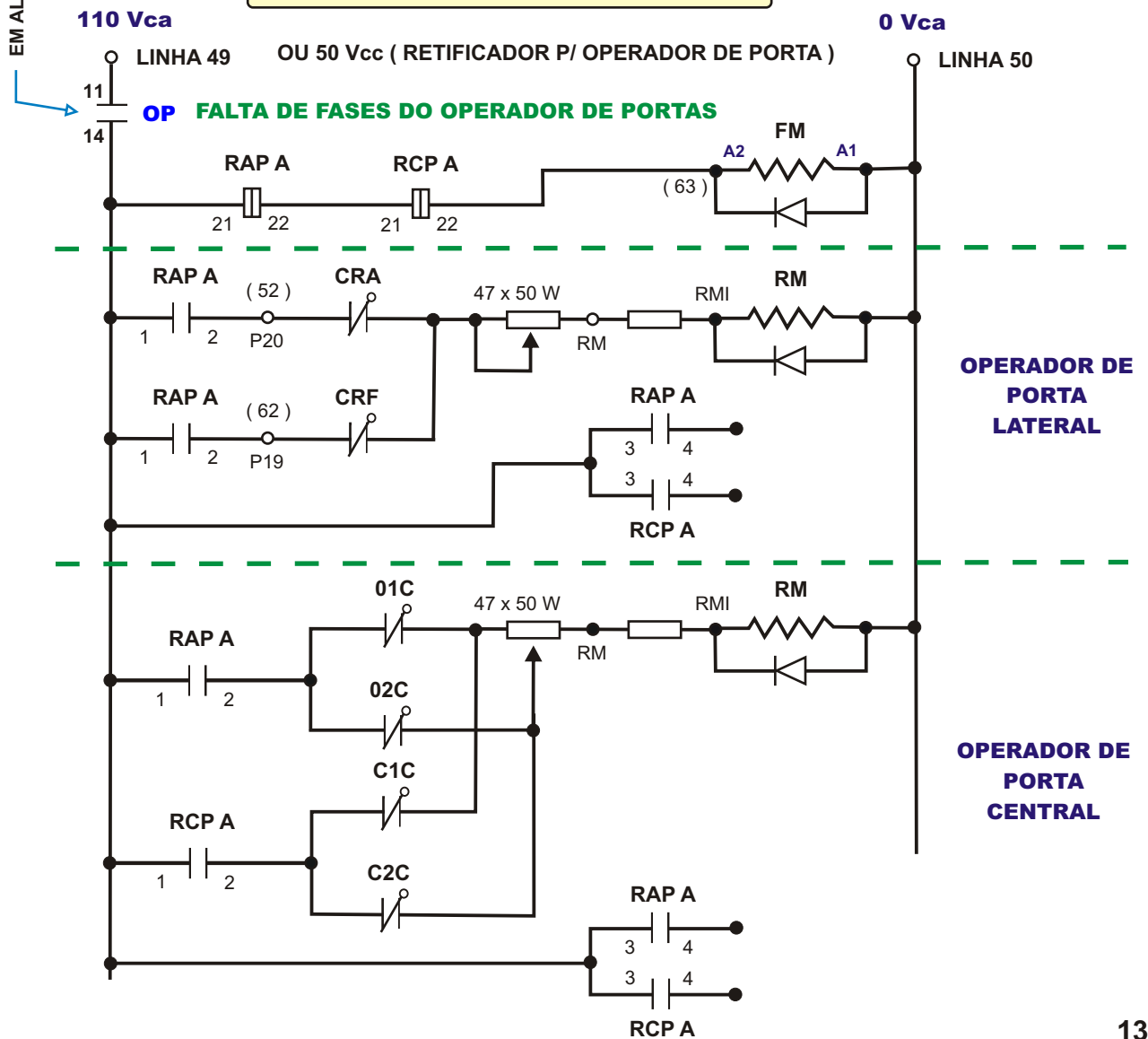
CIRCUITO PARA OPERADOR DE PORTA SÛR
