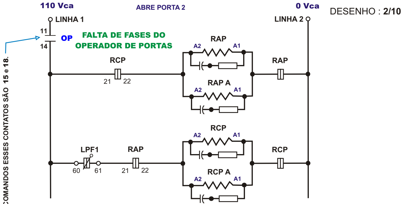
CIRCUITO PARA OPERADOR DE PORTA SÛR
