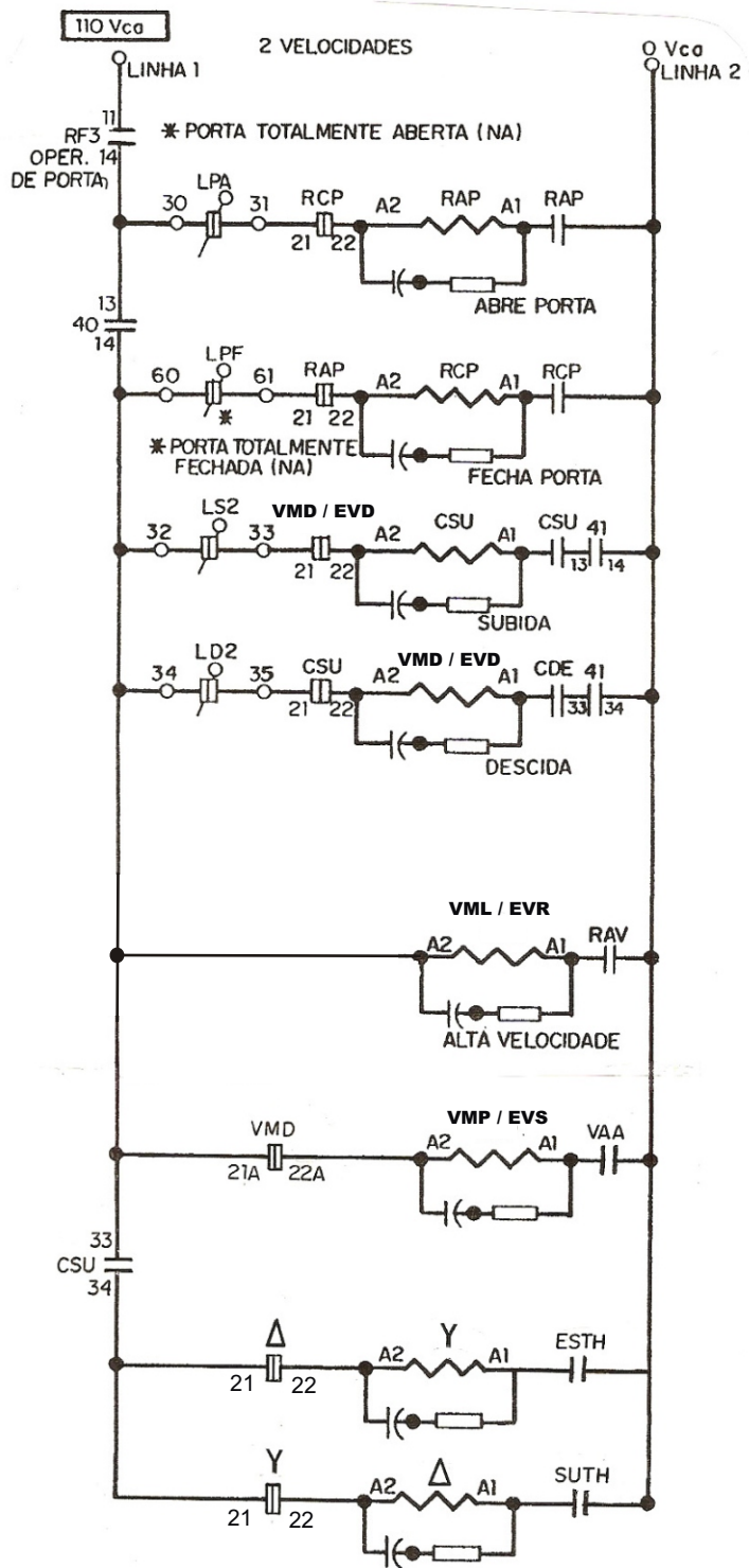
Diagrama Elétrico do Bloco de Válvulas
